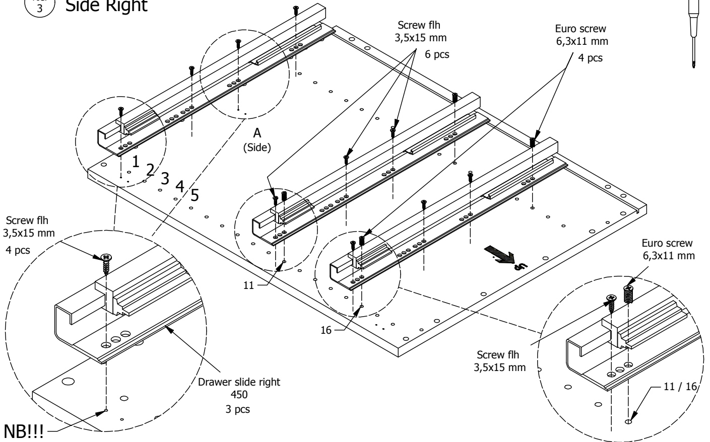
FIG. 4 Side Right
