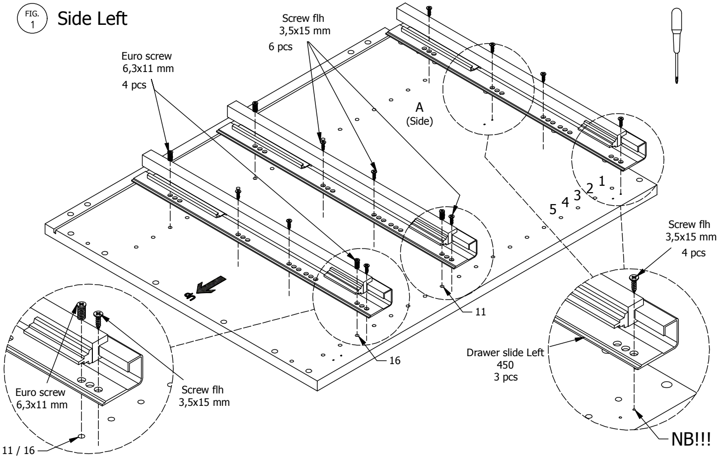
FIG. 2 Side Left
