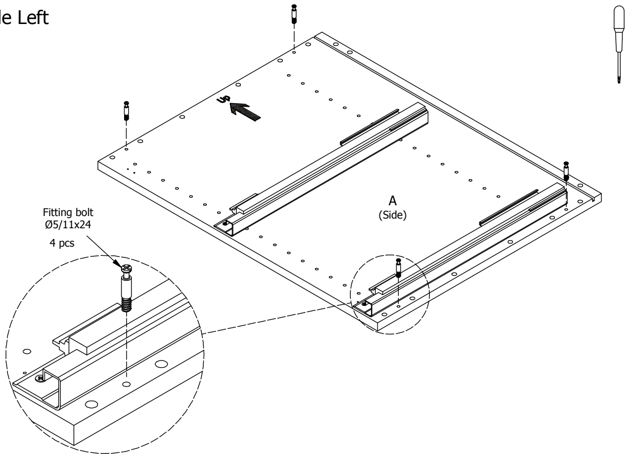
FIG. 4 Side Right
