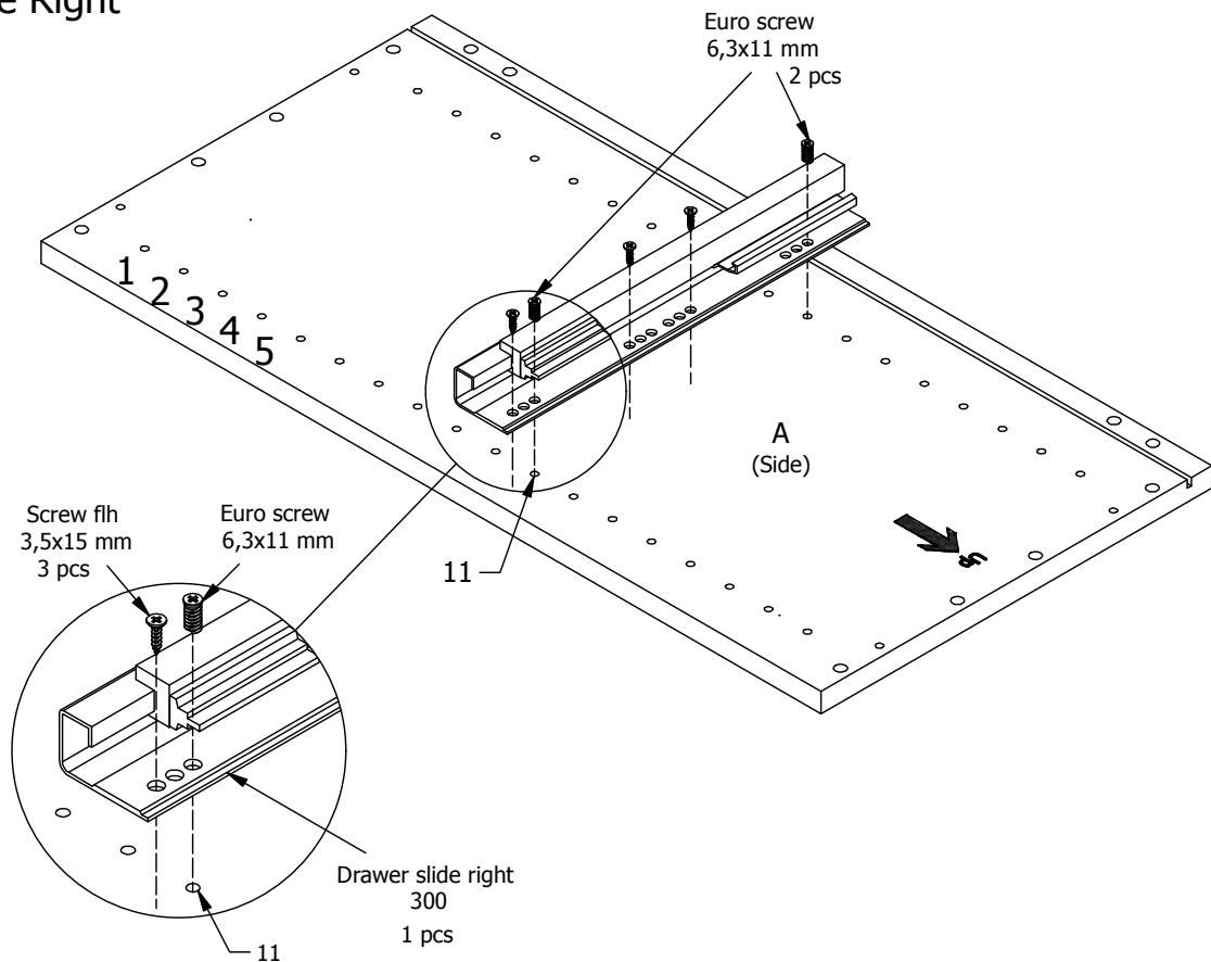
FIG. 2 Side Right
