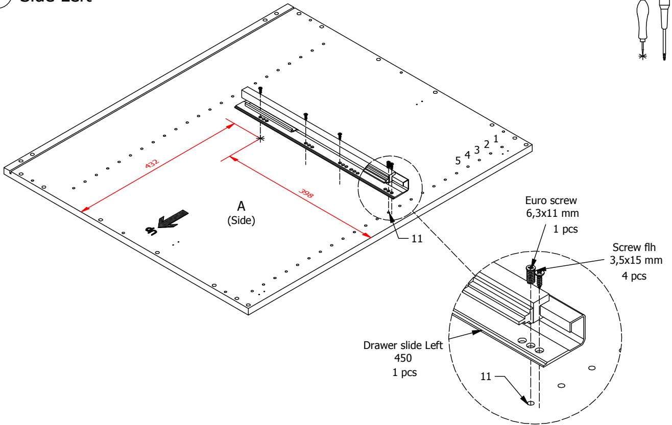
FIG. 1 Side Left
