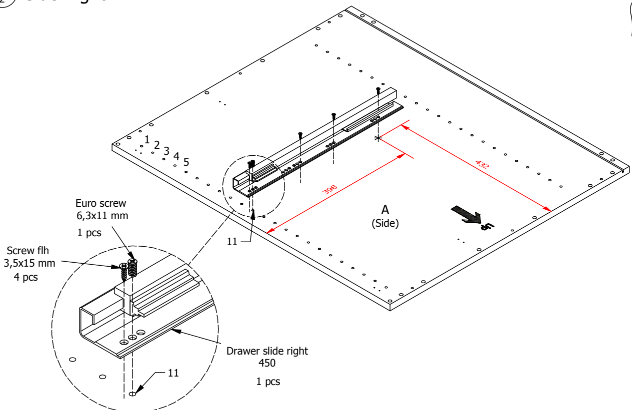
FIG. 2 Side Right
