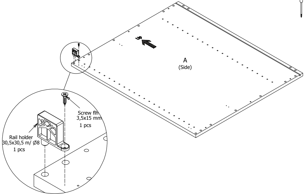
FIG. 2 Side Right
