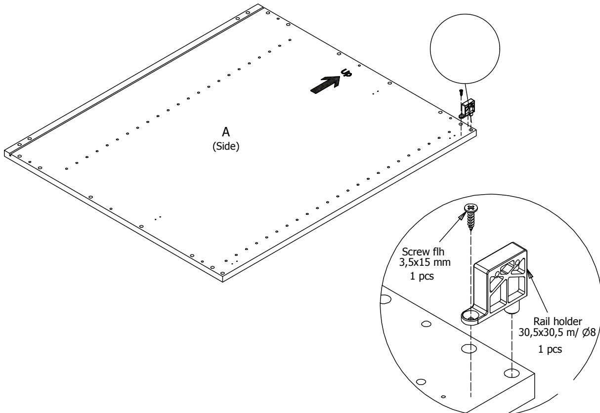
FIG. 2 Side Right
