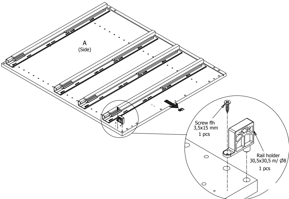
FIG. 6 Side Right
