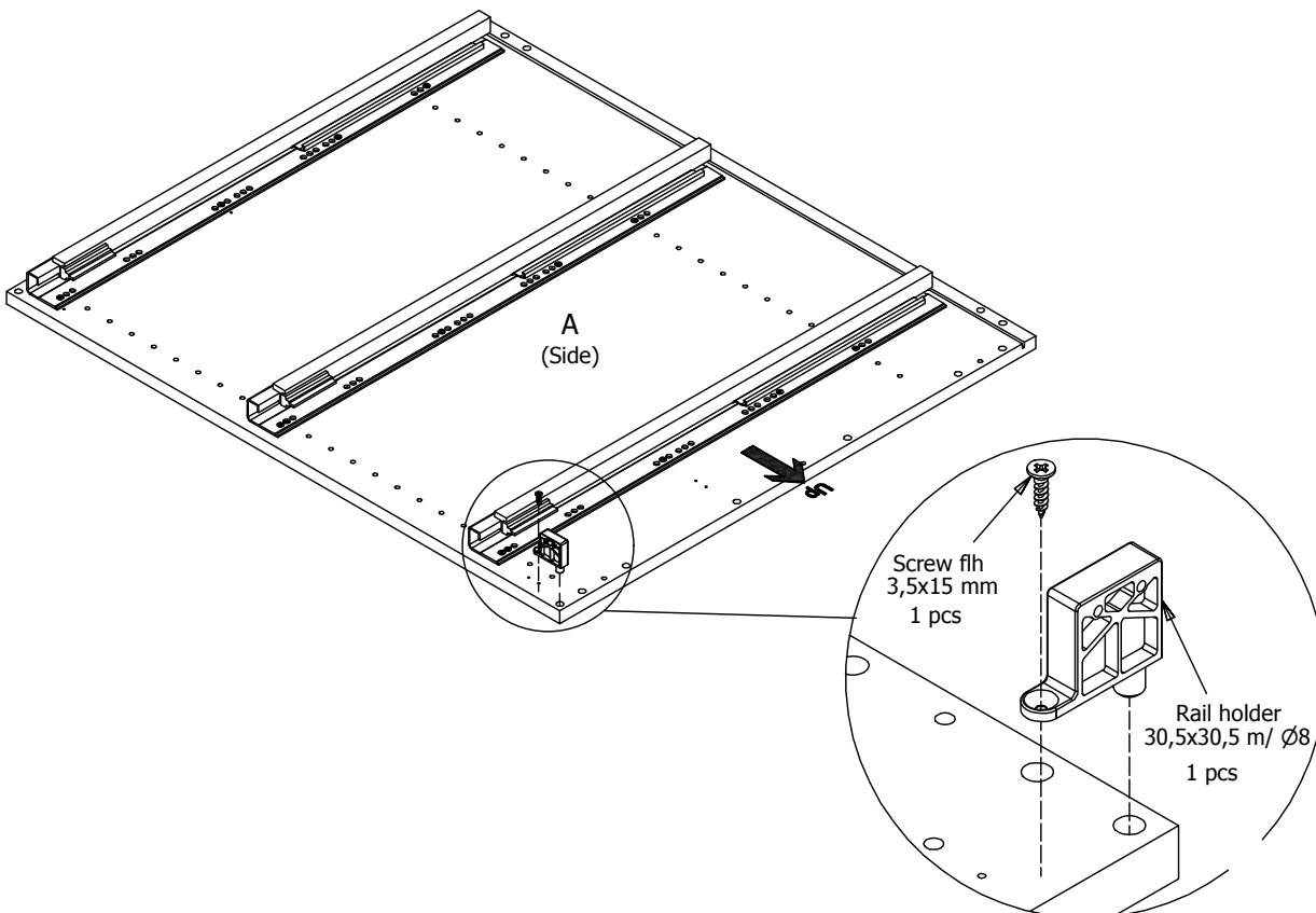
FIG. 6 Side Right
