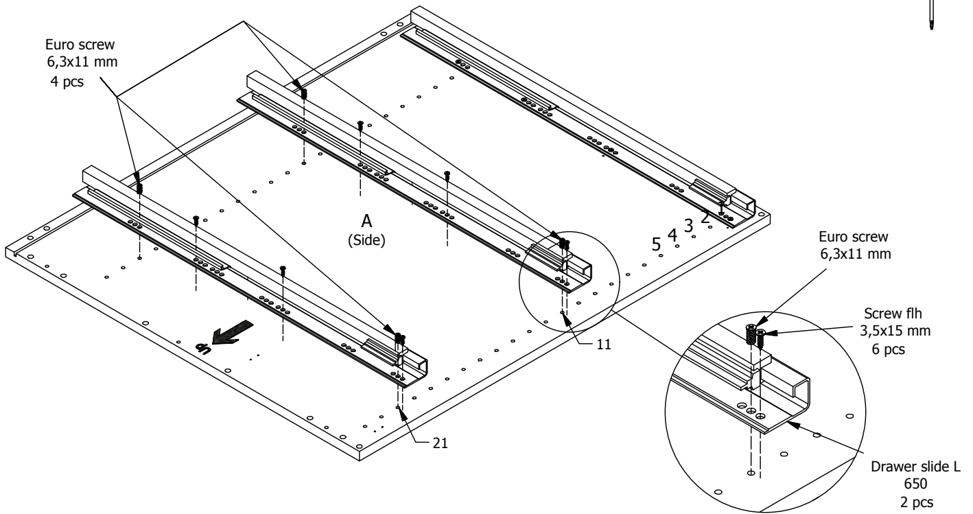
FIG. 4 Side Right
