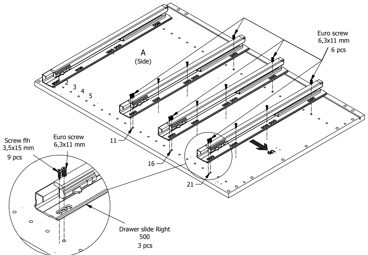
FIG. 4 Side Right
