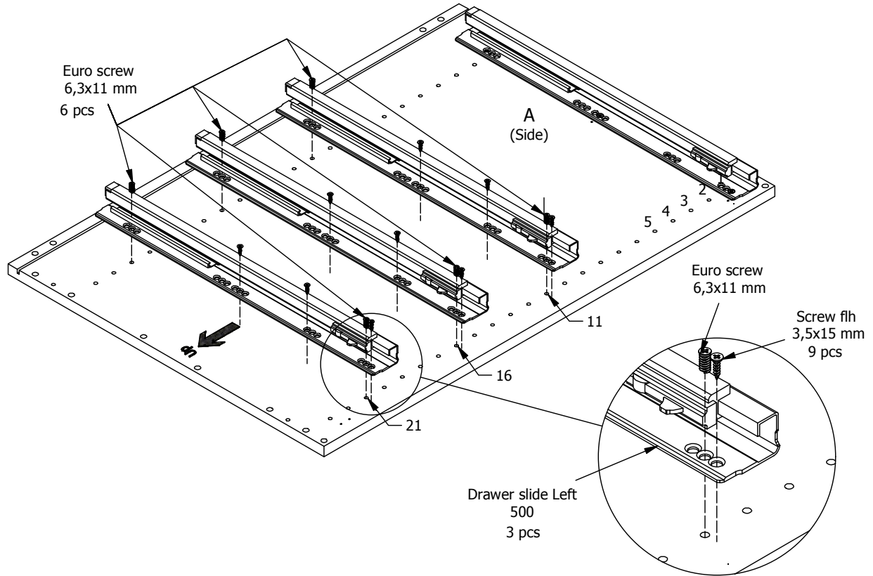
FIG. 3 Side Left
