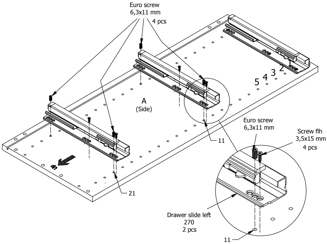
FIG. 3 Side Left
