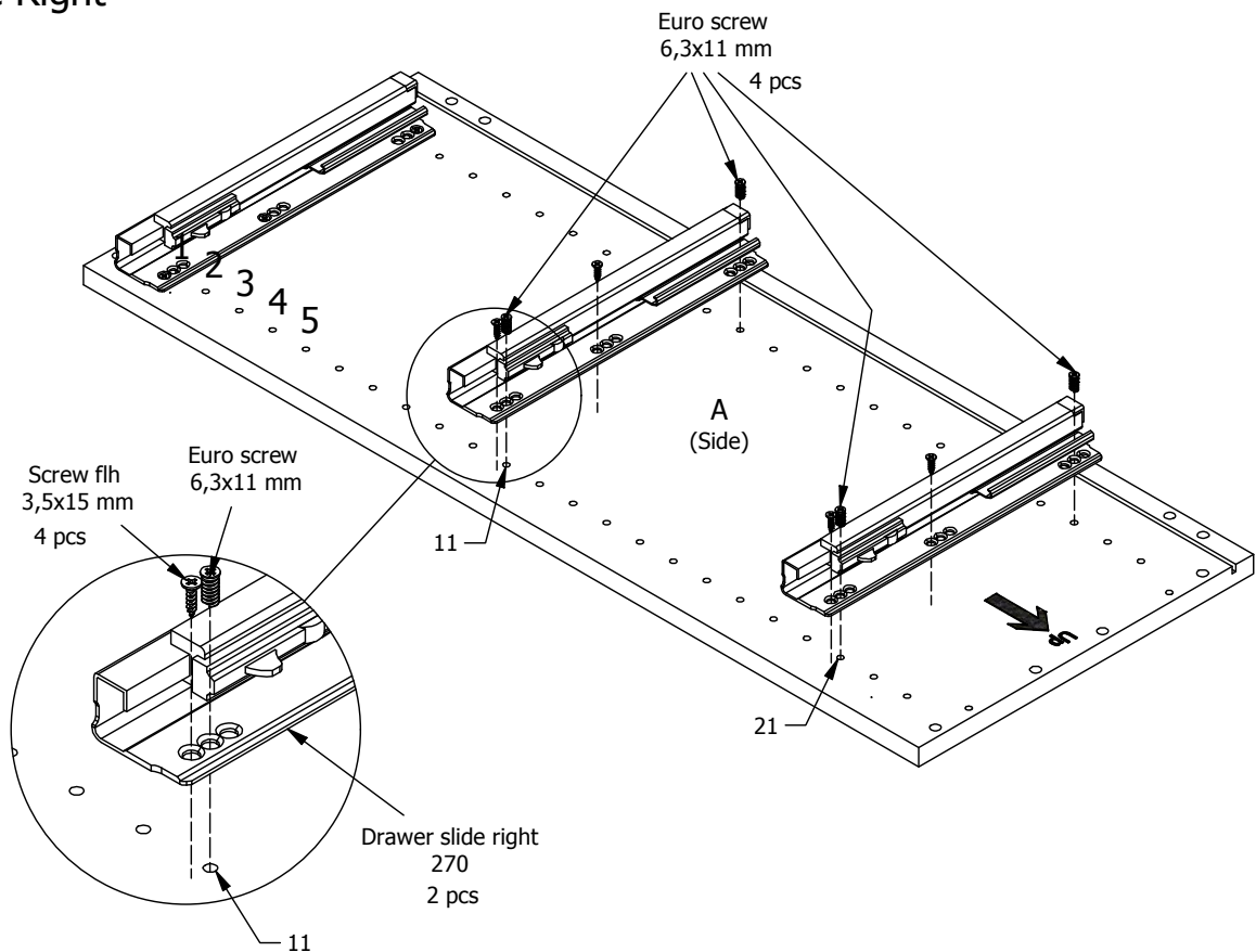
FIG. 4 Side Right
