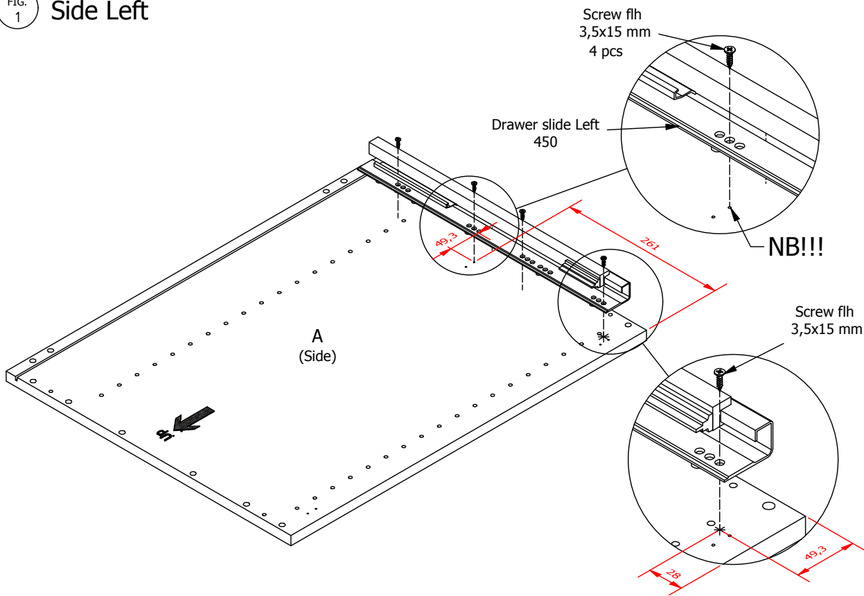
FIG. 2 Side Left
